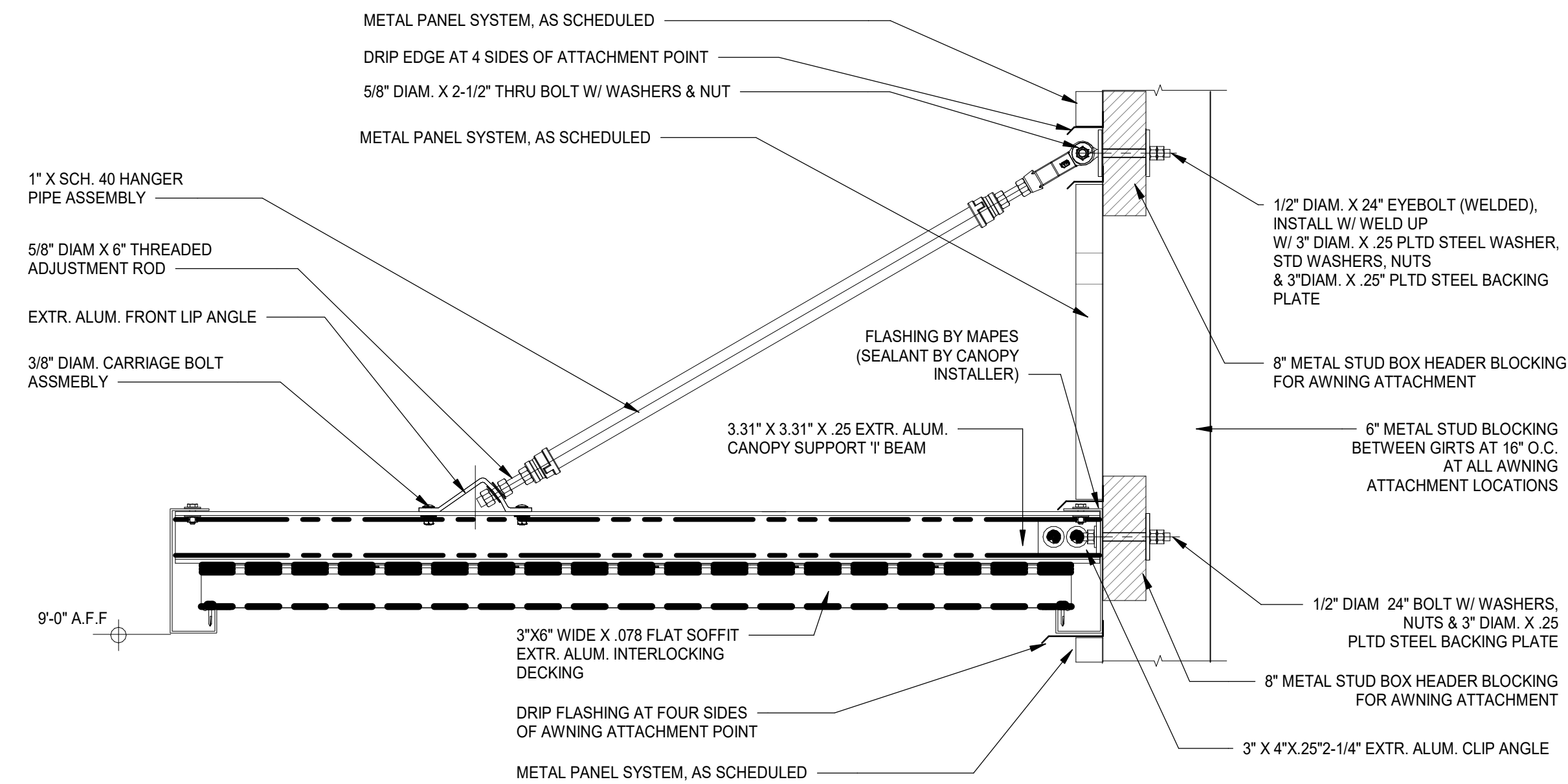
11 A50-03 METAL CANOPY SCALE: 1 1/2" = 1'-0"
