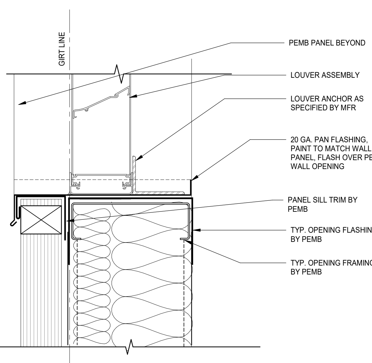
12 LOUVER SILL SCALE: 3" = 1'-0"
