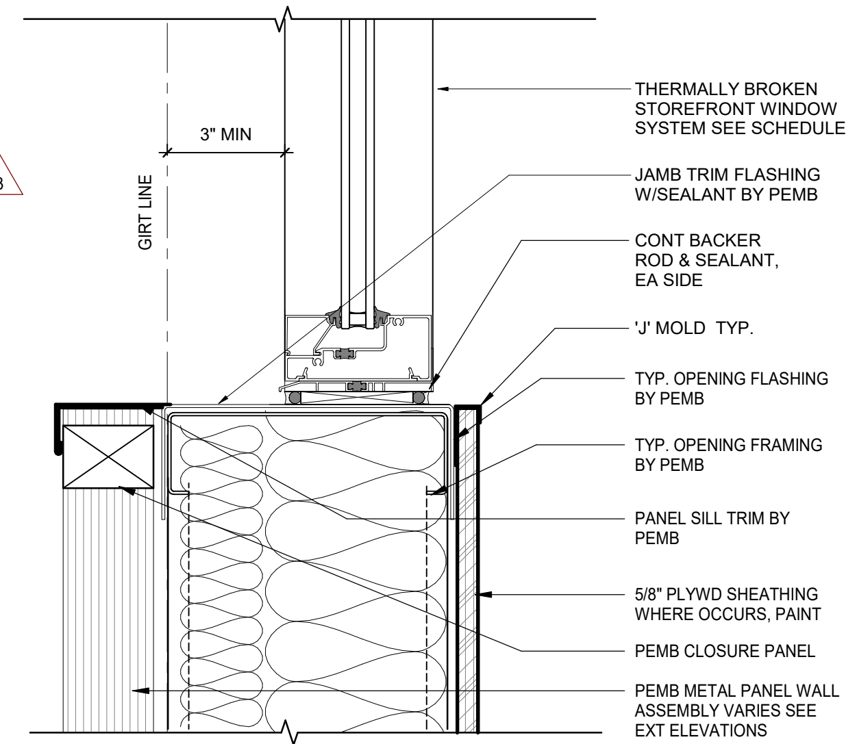
8 WINDOW SILL @ PEMB SCALE: 3" = 1'-0"
