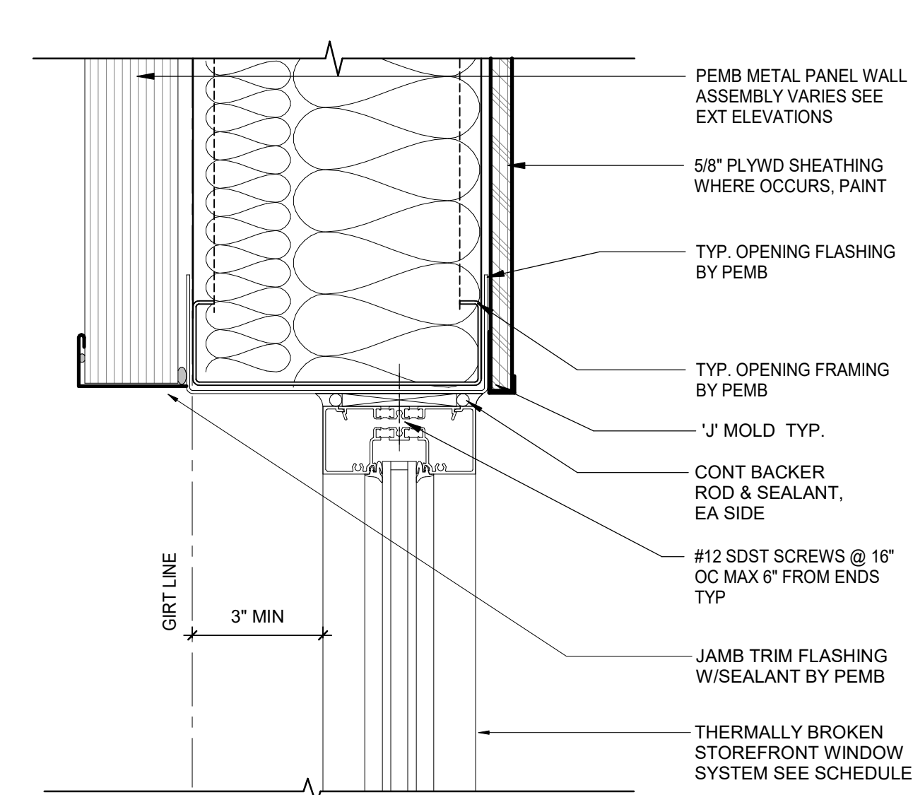
7 WINDOW JAMB SCALE: 3" = 1'-0"
