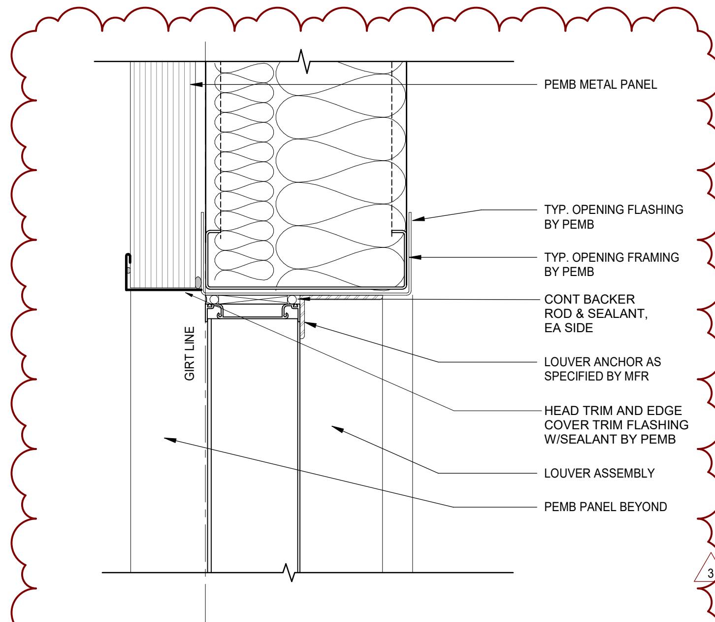
10 LOUVER JAMB SCALE: 3" = 1'-0"
