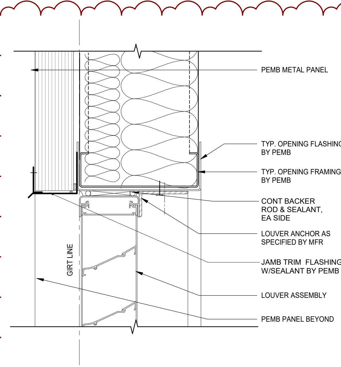
9 LOUVER HEAD SCALE: 3" = 1'-0"
